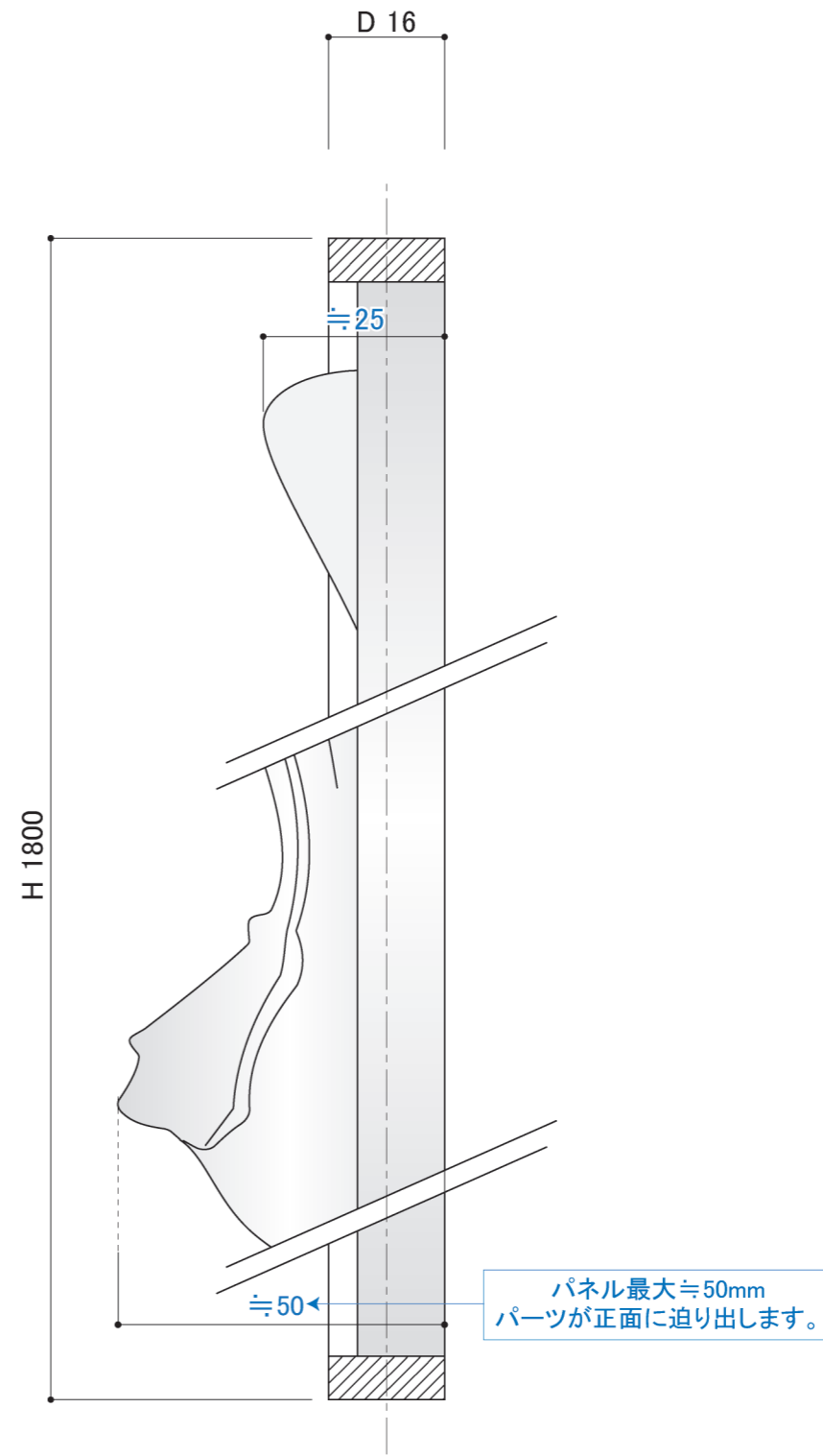
〈側断面詳細図 S=1/1〉
