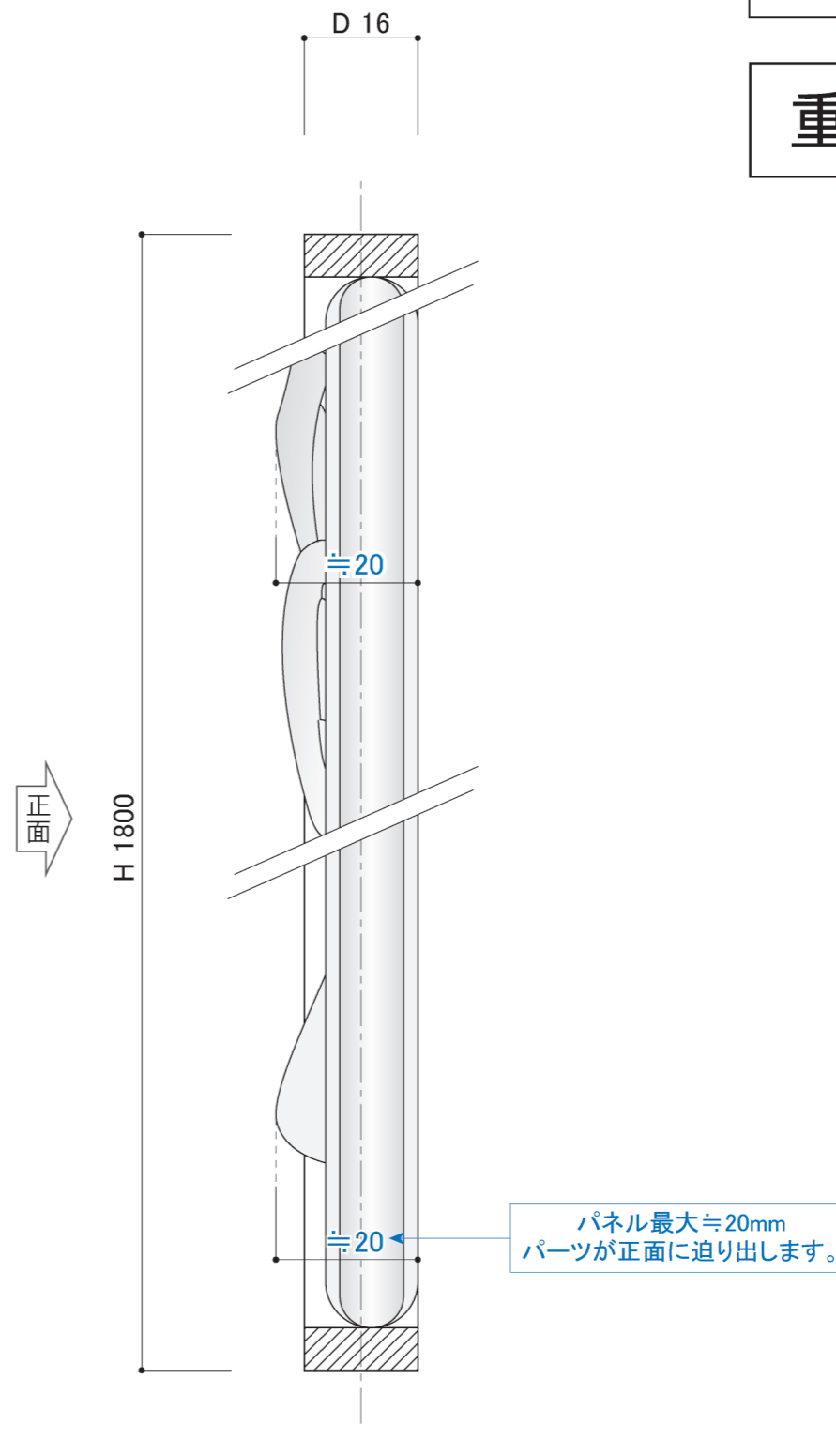
〈側断面詳細図 S=1/1〉
