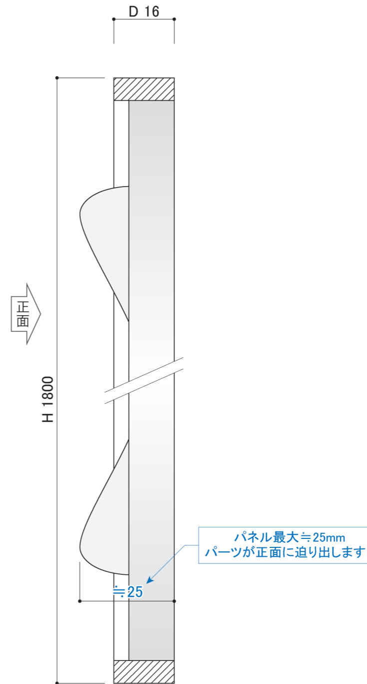
〈側断面詳細図 S=1/1〉
