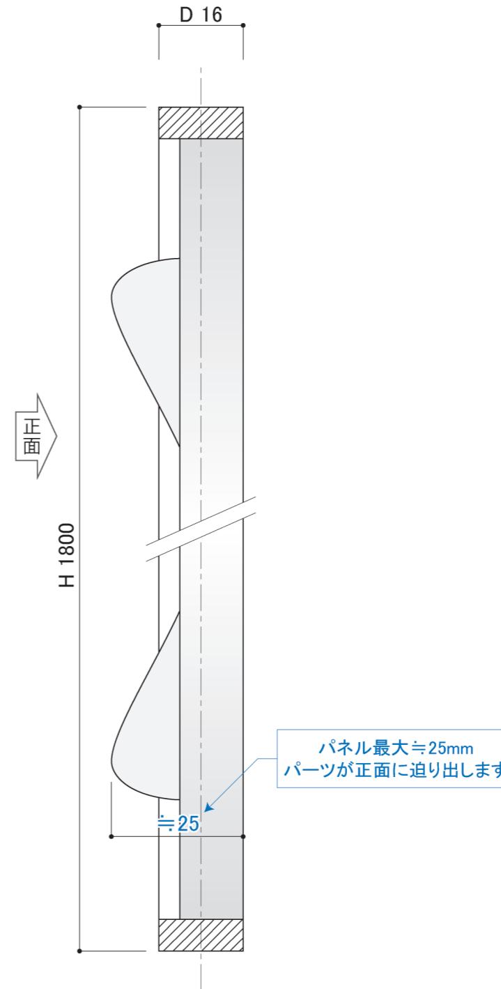
〈側断面詳細図 S=1/1〉
